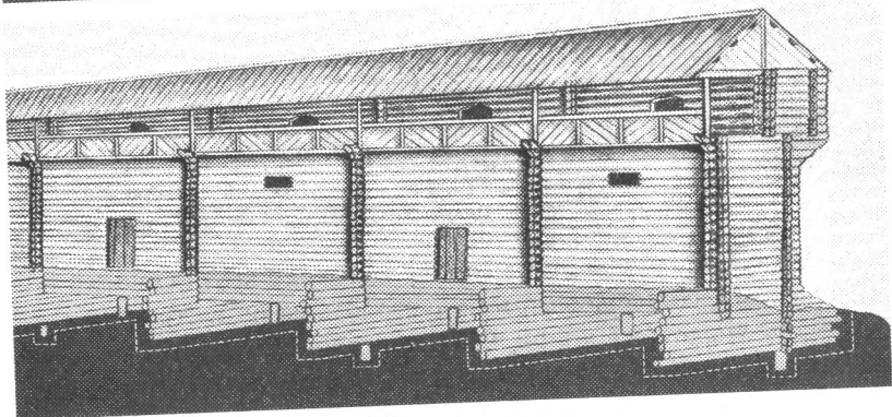
Тарасная стена Томского кремля. Внешний и внутренний фасады. Реконструкция и рисунок М. П. Черной
